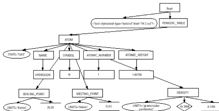
图 14-1 以树形图表示的清单 14-1
