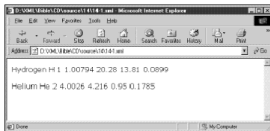
图 14-3 将清单 14-4 中调整过的 XSL 样式单应用于清单 14-1 中的 XML 文档，在 Internet Explorer 5.0 中生成的页面
