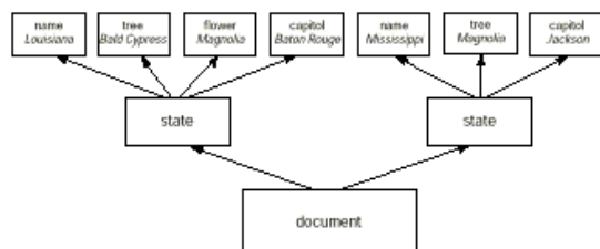
图 6-1 清单 6-1 表示的树形结构
