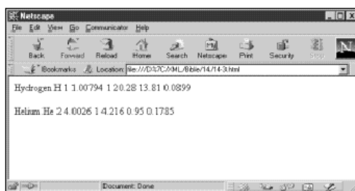
图 14-2 将清单 14-2 中的 XSL 样式单应用于清单 14-1 中的 XML 而生成的页面
